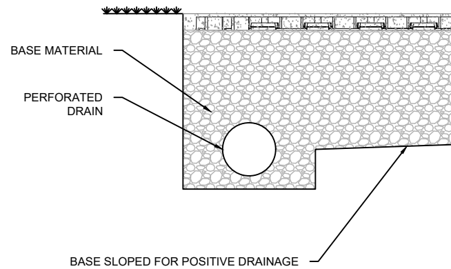
OPTIONAL UNDERDRAIN
